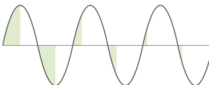
➤ Figuur 2: dimmen met fase-afsnijding
